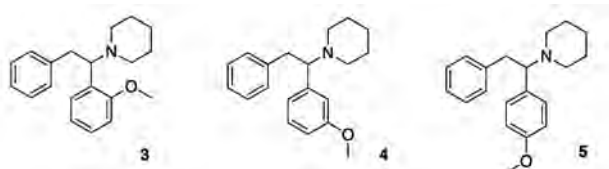
Obrázek 2: Strukturální vzorce konstitučních izomerů methoxfenidinu (2-MXP (3), 3-MXP (4) a 4-MXP (5))
