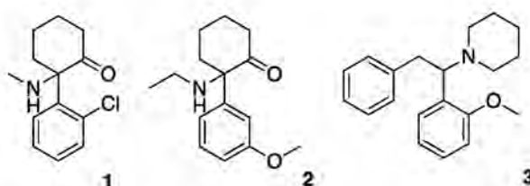
Obrázek 1: Strukturální vzorce ketaminu (1), methoxetaminu (2) a methoxfenidinu (3)
