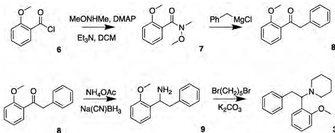
Schéma 1: Syntéza methoxfenidinu (3) 19
