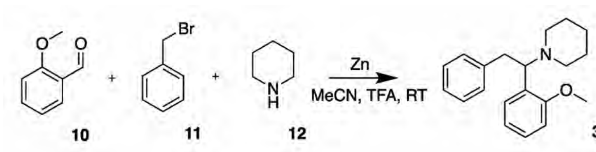
Schéma 2: One pot syntéza methoxfenidinu (3) 19
