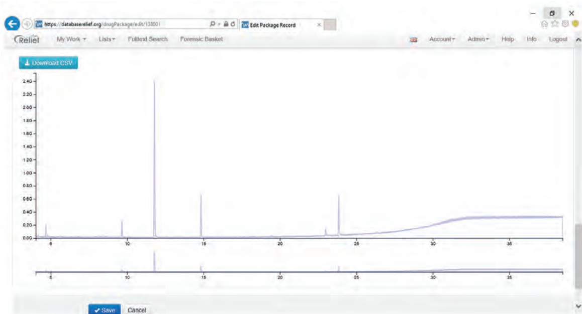
Obr. 5: Chromatogram (Zdroj: NPC)
